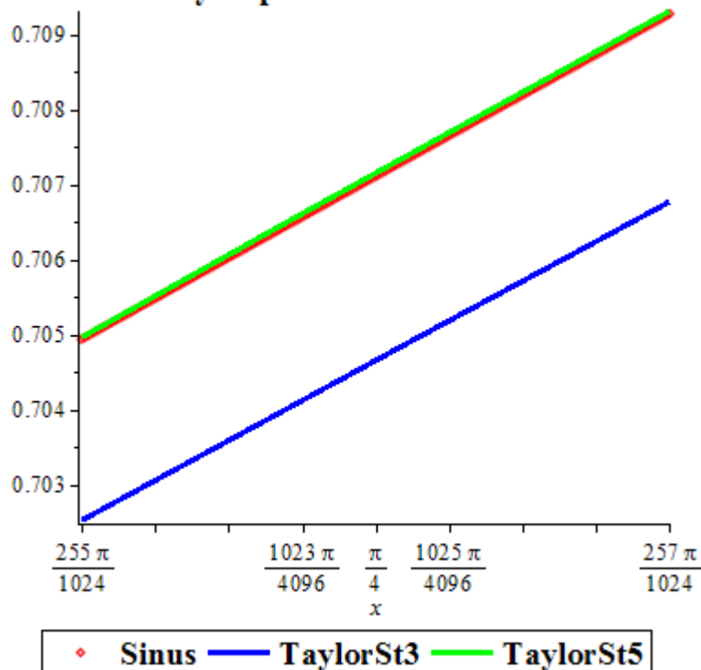
Taylor pro sinus v okolí \pi/4
