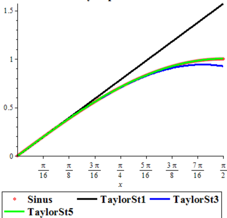
Taylor pro sinus
